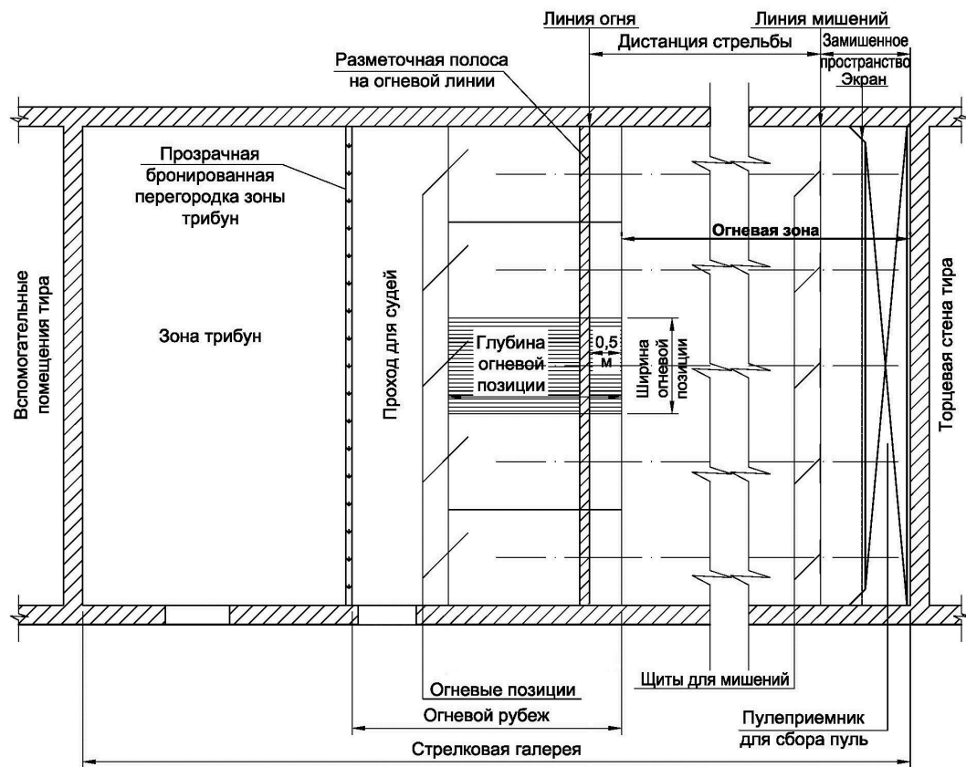
Рис.1. Стрелковая галерея.
