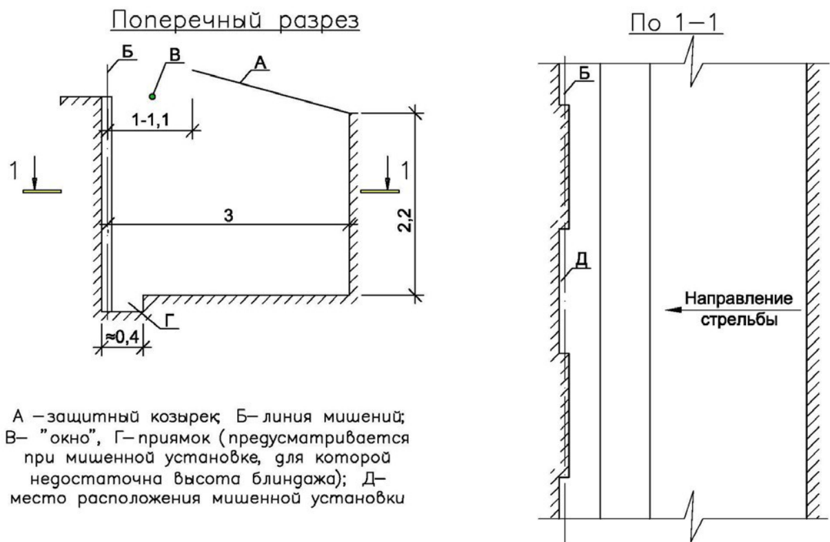
Рис. 2. Заглубленный блиндаж огневой зоны закрытого тира (размеры, м).
